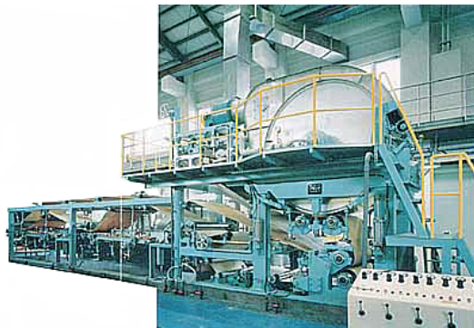
短網円網コンビネーションマシン
