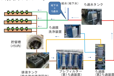
養液栽培用液肥循環システムの概要
